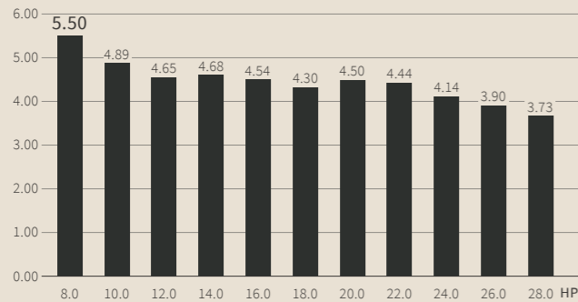
Cooling EER
